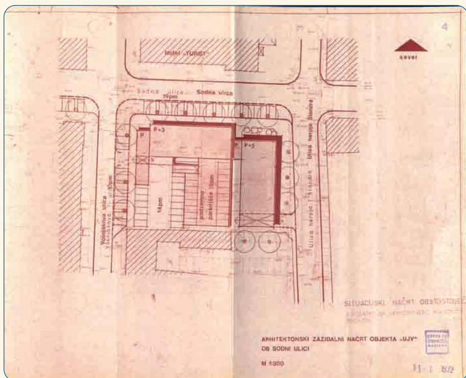
Slika 7: Zazidalni načrt objekta PM Maribor, 1972
