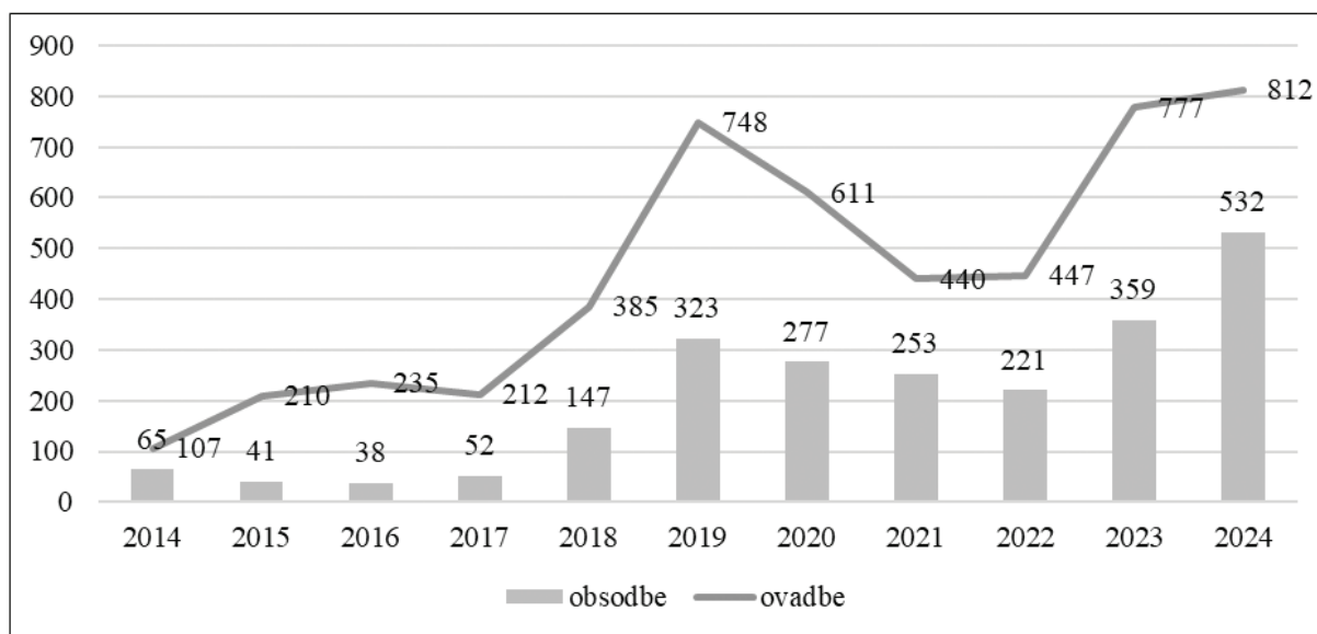
Graf 1: Ovadbe in obsodbe po 308. členu Kazenskega zakonika 2014–2024 (vir: Statistični urad Republike Slovenije [SURS], 2025)
