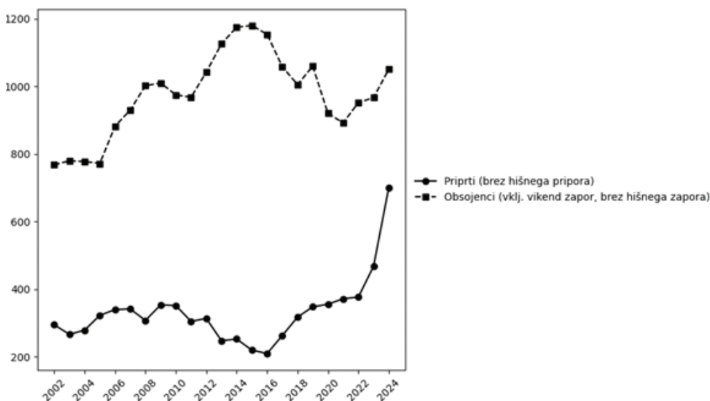
Graf 2: Povprečno število priprtih oseb in obsojencev v obdobju 2002–2024 (vir: URSIKS, 2025)
