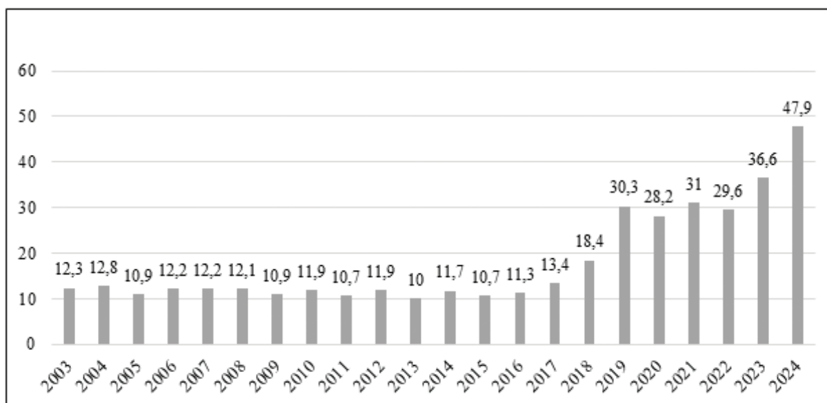
Graf 3: Delež tujcev med zaprtimi osebami (vir: URSIKS, 2025)
